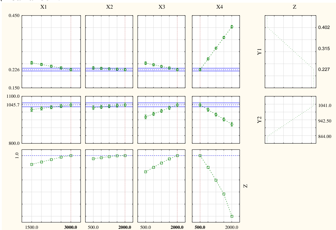
Рисунок 3 – Графічне відображення процедури знаходження оптимального складу композиційної присадки на основі геомодифікатора КГМТ-1
