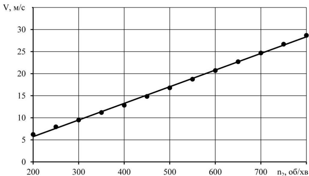
Рисунок 2 – Залежність загальної швидкості частинки V вороху від частоти обертання обчисуючого барабану n_2
