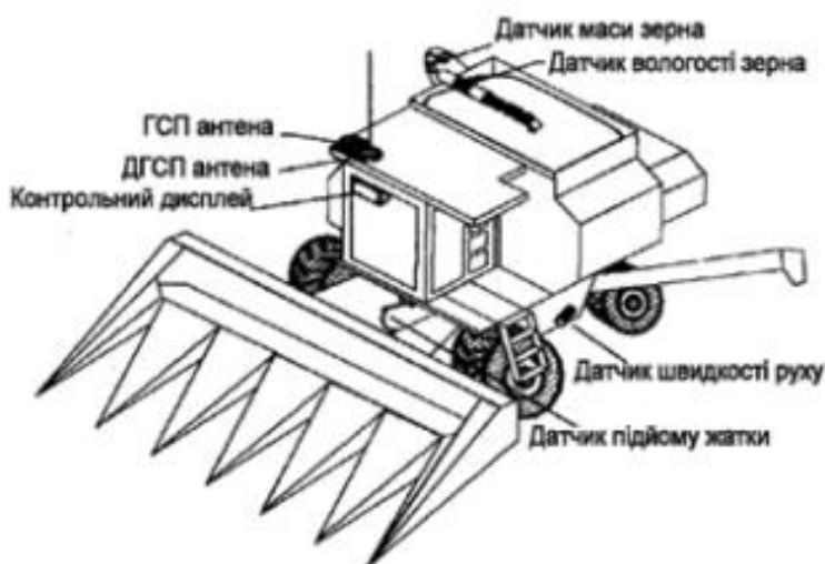
Рис. 1 - Комплект обладнання для картографування врожайності [0]
