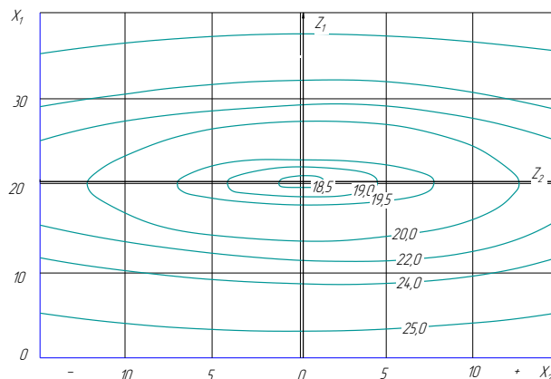
Рис. 3. Двовимірний переріз поверхні відгуку, що характеризує показники нерівномірності розподілу добрив за умови X_3 = 0 .
