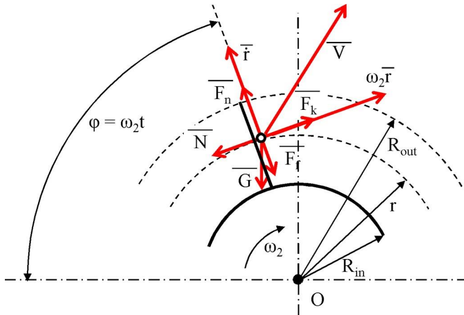
Рисунок 1 – Взаємодія частинки вороху з обчисуючою гребінкою
