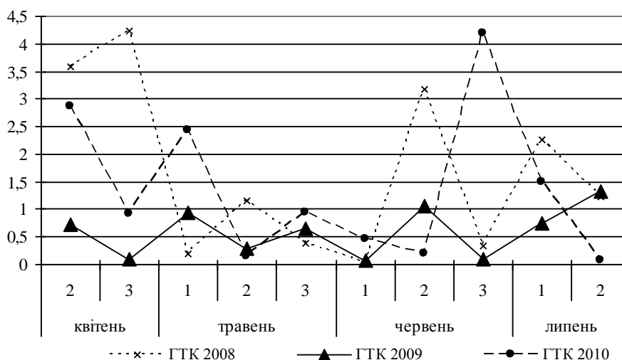
Рис. 1. Динаміка гідротермічного коефіцієнта Г. Т. Селянінова за вегетаційний період пшениці ярої (Дослідне поле ХНАУ, 2008-2010 рр.)
