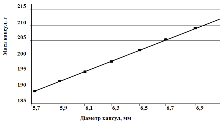
Рис. 13. Залежність маси 1000 шт. капсульованого насіння від діаметра
